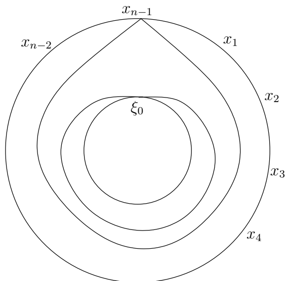
FIG. 5. (\xi_0)_{[-1]}(x_{n-1})_{[1]}
